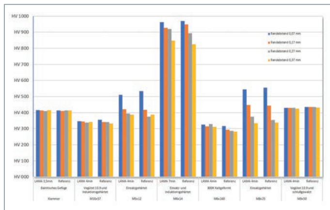
Abb. 5.2: Ergebnisse des Härte- und Korrosionstests
