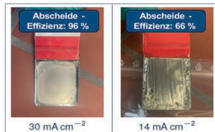
Abb. 3: Einfluss von Milchsäure (r.) auf die Effizienzen und Morphologien galvanostatischer Abscheidungen aus eisenchloridbasierten Elektrolyten. Das linke Bild zeigt eine Abscheidung ohne Milchsäure. Elektrolyte: 0,8M FeCl 2 + 3M NH 4 Cl, Additivkonzentration 1M; Abscheidebedingungen: pH = 3,5 (mit Ammoniak eingestellt), RT, mit Rührung
